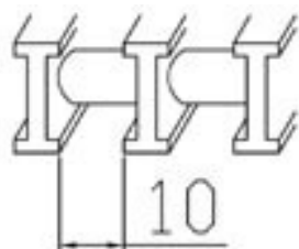
AluRoll/Fix250/10
